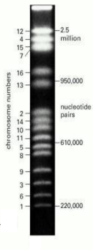
S.cerevisiae chromosomes on a CHEF gel
