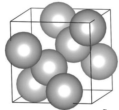
Mg sublattice
