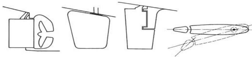
Simplex rudder
