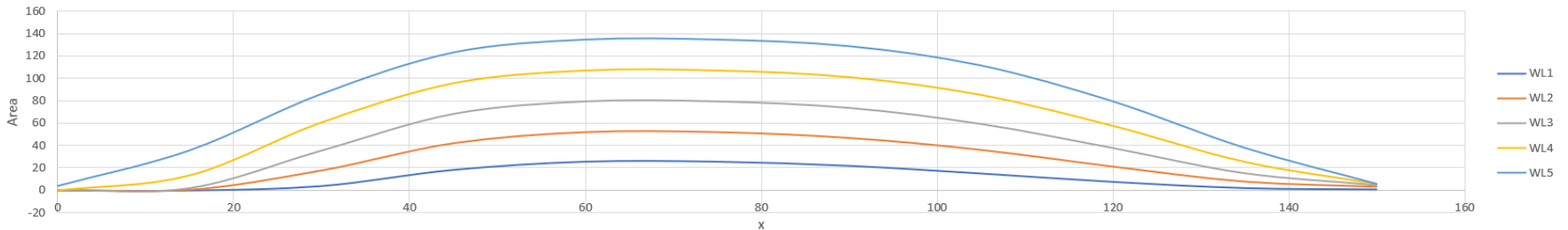
SACs
