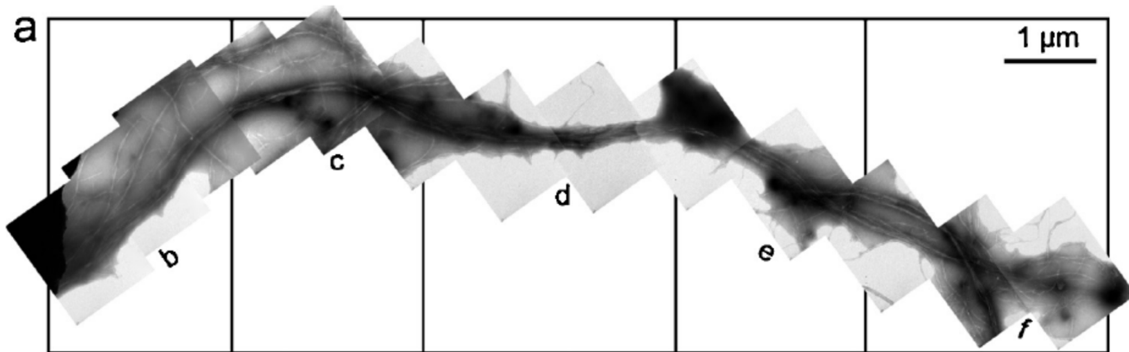
String of TEM images of a 12.7 μm long cellulose nanofibril
