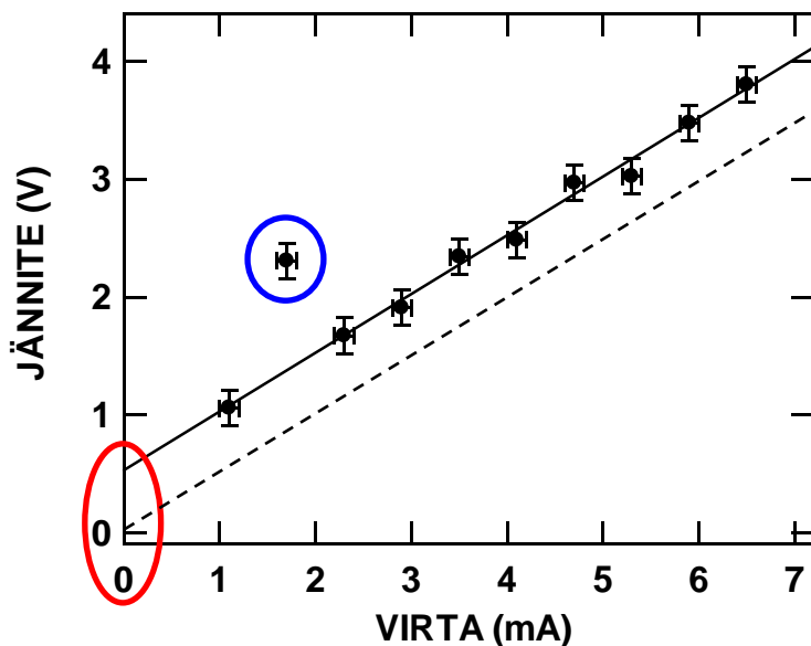
Kuva 1. Erilaiset virhetyyppejä havainnollistava mittaus. Yksi mittaustuloksista voidaan luokitella karkeaksi virheeksi (sininen), mittauksessa esiintyy myös systemaattista virhettä (punainen), sillä se poikkeaa teoreettisesta riippuvuudesta (katkoviiva). Satunnaisvirhettä taas kuvaa mittauspisteiden poikkeamat sovitetulta suoralta (yhtenäinen viiva).
