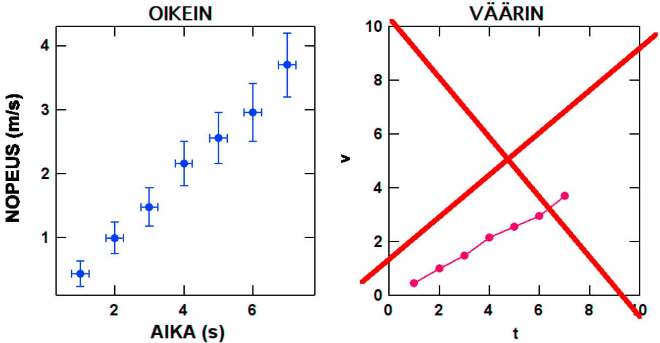
Kuva 6. Mitattujen pisteerien (x,y) sekä niiden virherajojen sijoittaminen koordinaatistoon. Vasemmanpuolisessa kuvassa asteikko on valittu siten, että koko kuva-ala täyttyy. Oikeanpuoleisesta kuvasta puuttuvat yksiköt asteikoilta sekä pisteiden virherajat. Asteikot on valittu huonosti ja pisteet on yhdistetty murtoviivalla.
