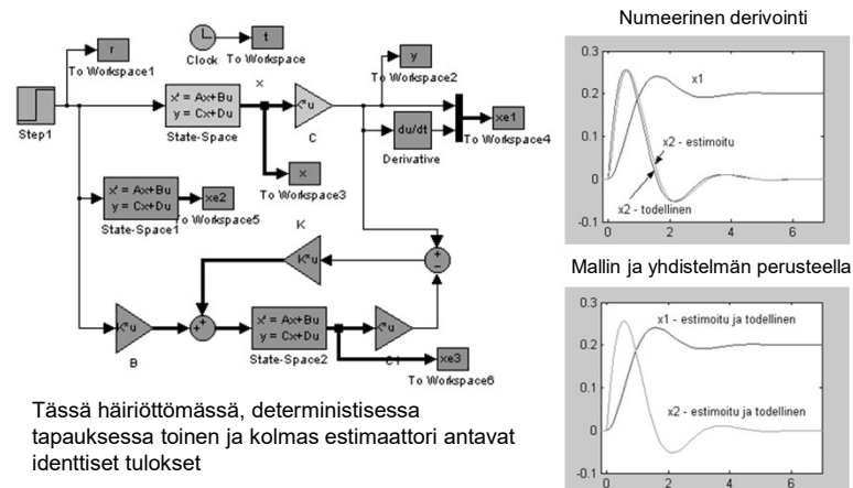
Numeerinen derivointi
