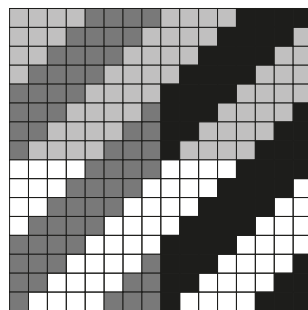
I / A 4:4 TWILL
