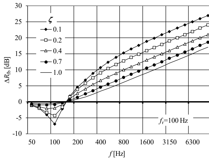
Kuva 5.12.2 Joustavan rangan tuottama lisäeristys \Delta R_{fb} kaksinkertaisen levyrakenteen kytkennän kautta muodostuvaan ilmaaneneristävyteen vaimennussuhteen \zeta eri arvoilla, kun resonanssitaajuus f_r on vakio.
