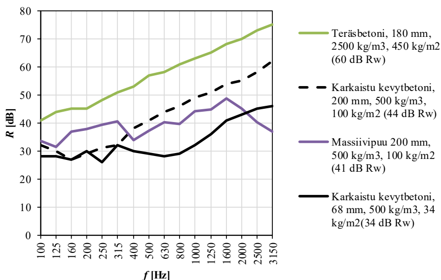
Kuva 5.10.2 Raskaiden rakenteiden ilmapääneneristävyyksiä taajuuden funktiona. Sulkeissa R_w .
