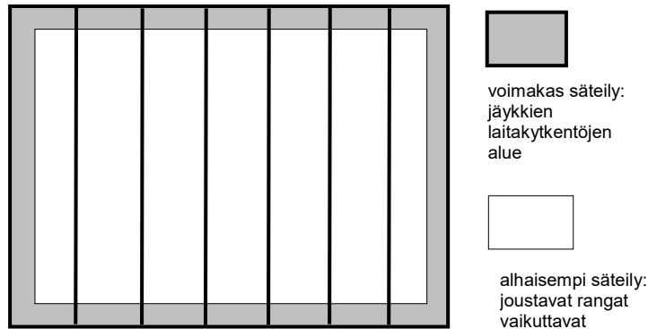
Kuva 5.12.3 Joustavilla rangoilla toteutetun kaksinkertaisen levyrakenneseinän ilmasteneristävyyden heikkenee, jos laidoilla on jäykkiä kytkentöjä.
