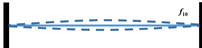
Kuva 5.5.1 Alin ominaistaajuus f_{10} , jossa levy värähtelee kokonaisuudessaan sen kiinnityspisteiden suhteen levyn pisimmässä suunnassa.
