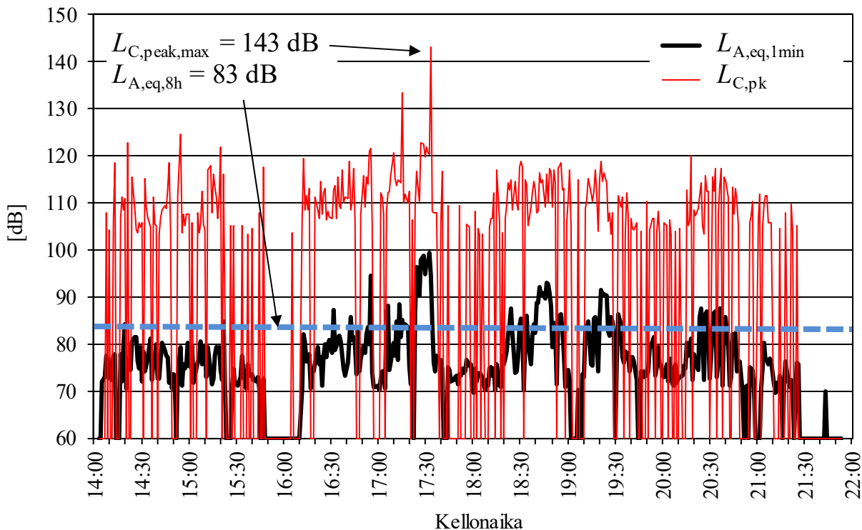
Kuva 9.1.1. Meluallistusta mitataan työpaikoilla meluannosmittarilla, joka koostuu korvan läheisyyteen sijoitettavasta mikrofonista sekä taskuun sopivasta tallentimesta. Käyrä esittää suureen L_{p,A,eq,1min} arvoja ajan funktiona. Mittausajalta määritetään vähintään ekvivalenttitaso L_{p,A,eq} sekä huippuäänitaso L_{C,peak,max} .
