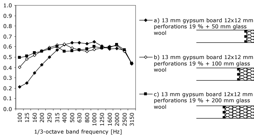
Kuva 3.7.2 Rei'itetyn 13 mm paksun kipsilevyn normaalin tulokulman absorptiosuhteen riippuvuus kaviteetin paksuudesta (0, 50, 100 ja 200 mm), kun (a) kaviteetti on tyhjä tai (b) kaviteetti on täytetty mineraalivillalla ( \rho=18 \text{ kg/m}^3 , r=9600 \text{ Pa}\cdot\text{s/m}^2 ). Kummassakin kuvassa kipsilevyn takapinnassa oli tuotteen mukainen huopa ( R_s=1183 \text{ Pas/m} ). Reikäsuhde on \varepsilon=0.19 .
