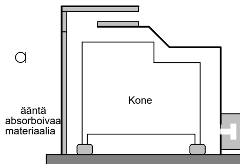
Kuva 10.6.2. Tyypillisesti saavutettavia melunvaimennuksia erilaisilla koneen ja koteloinnin järjestelyillä.
