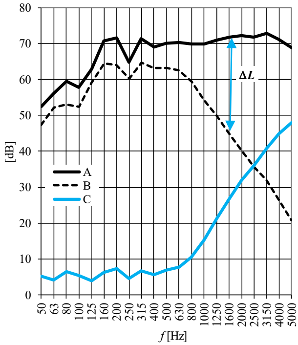
Kuva 6.4.1 Erään lattiapäällysteen askeläänenparannusluvun testaustulos.
