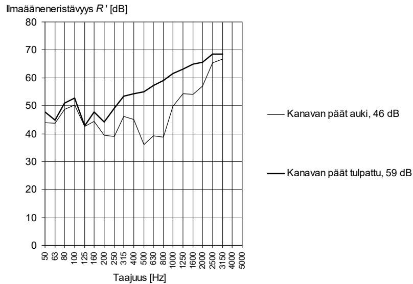
Kuva 8.9.2. Mittaustulos asuinhuoneistojen välillä, jossa ilmanvaihtokanaviston kautta tapahtuva sivutiesiirtymä heikensi rakenteiden sallimaa ilmaääneneristyslukua 13 dB.
