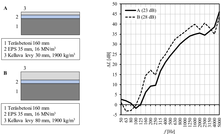
Kuva 6.5.2 Esimerkki kahden toisistaan hieman poikkeavan kelluvan lattiarakenteen tuomasta askeläänepainetason parannuksesta \Delta L raakaväliopajaan (1) nähden. \Delta L_w -arvot ovat sulkeissa.
