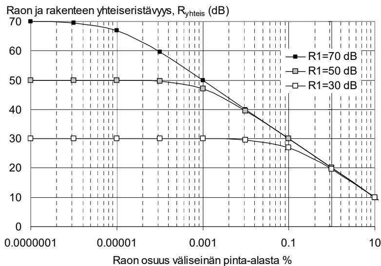
Kuva 8.7.2. Raon ja rakenteen yhteiseristävyys erilaisilla raon pinta-aloilla, kun tiiviin rakenteen ilmääneneristävyys on 30, 50 tai 70 dB. Esimerkiksi 10 m 2 kokoisessa rakenteessa 0.0001 % tarkoittaa 1x10 mm kokoista rakoja.
