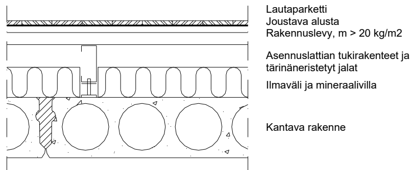
Kuva 6.8.1 Asennuslattian rakenneperiaate. (Lähde: RIL 243-1:2007)
