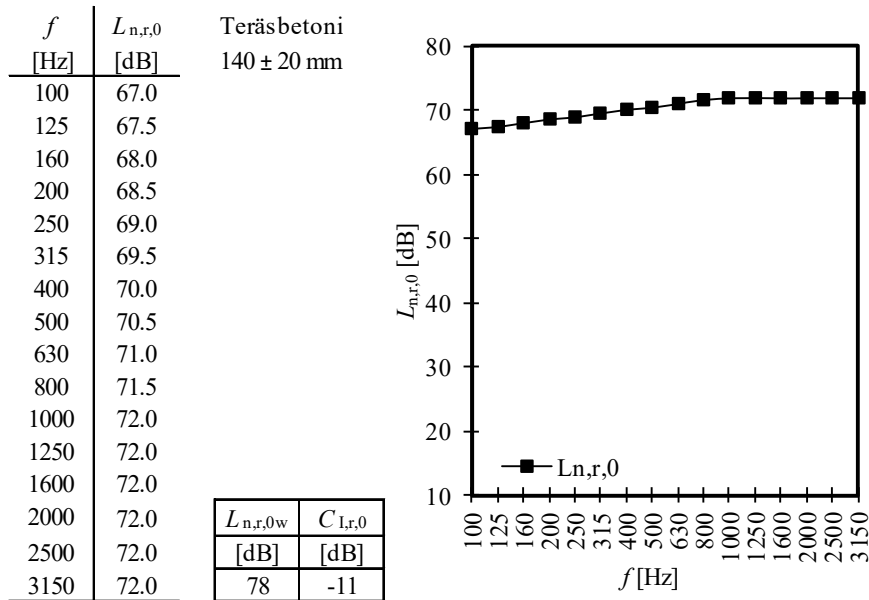
Kuva 6.3.1 Standardinmukaiselta referenssilattialta odotettu askeläänenpainetaso ISO 10140-5 (2010) mukaan.
