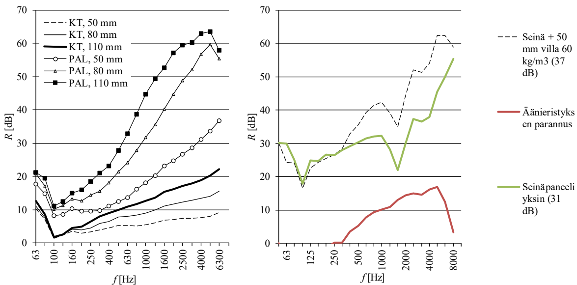
Kuva 5.14.1 (a) Lasivillan ilmasteneristävyys paksuuden ja tiheyden funktiona. PAL: \rho=117 \text{ kg/m}^3 , r=90\,000 \text{ Pa}\cdot\text{s/m}^2 . KT: \rho=19 \text{ kg/m}^3 ja r=8\,000 \text{ Pa}\cdot\text{s/m}^2 . (Hongisto et al., 2002) (b) 50 mm paksun mineraalivillalevytyksen vaikutus seinäpaneelin ilmasteneristävyyteen. Sulkeissa on esitetty R_w -arvot. Absorptiopinnoitus paransi ilmasteneristystä lähinnä 200 Hz:n yläpuolella. Vastaava parannus on havaittu myös massiiviseinän päälle asennetulla absorptiolevypinnoituksella. (RIL 243-1-2007)
