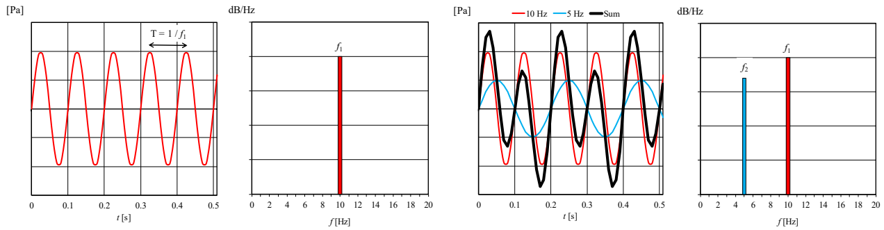
Kuva 1.4.1 (Yläriivi) Harmonisen siniaallon (10 Hz) äänenpaine ajan funktiona ja äänenpainetaso taajuuden funktiona. (Alarivi) Kaksi amplitudiltaan ja taajuudeltaan erilaista siniaalloa ja niiden summa.
