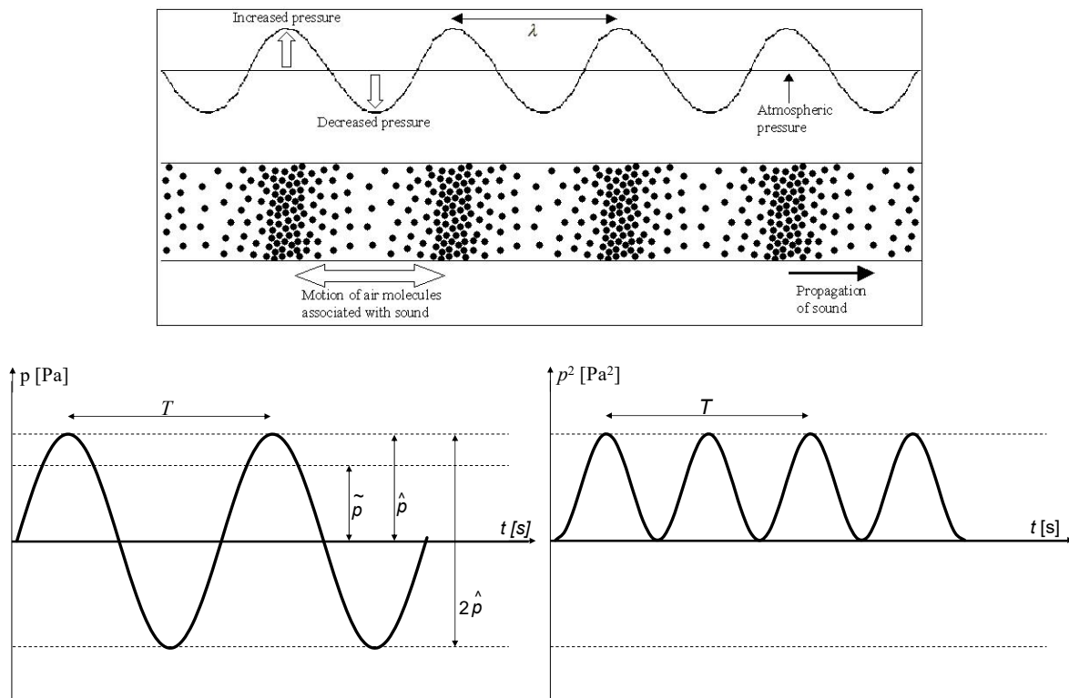
Kuva 1.1.1 (a) Ilmassa etenevä ääni on pitkittäistä aaltoliikettä eli puristus-aaltoliikettä ( longitudinal or compression wave ). Lähde: medium.com. Pitkittäistä aaltoliikettä esitetään graafisesti kuitenkin samoin kuin poikittaista aaltoliikettä ( transverse wave ) (Oliva, 2005). (b) Harmonisen, yhdellä taajuudella tapahtuvan äänisignaalin äänenpaine ajan funktiona ja siitä johdettava huippuarvo ( \hat{p} ), tehollisarvo ( \tilde{p} ) ja jakso T . Tässä kurssissa käsitellään ainoastaan harmonisia signaaleja eli signaaleja, jotka voidaan muodostaa sinimäisten aaltojen summana. (c). Edellisen neliö.
