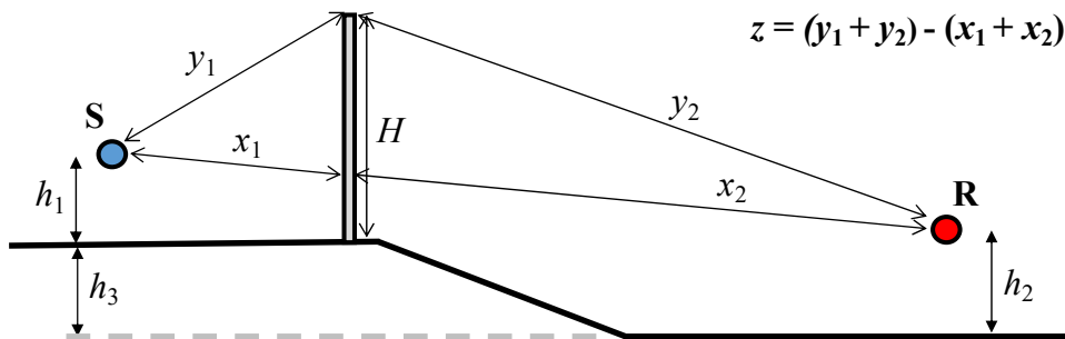
Kuva 2.9.1. Meluesteen matkaero z on meluesteen yli taittuvan äänireitin pituuden ( y_1+y_2 ) ja suoran äänireitin pituuden ( x_1+x_2 ) välinen erotus. Matkaero ratkaistaan trigonometrian avulla. S on äänilähde ja R on vastaanottaja.
