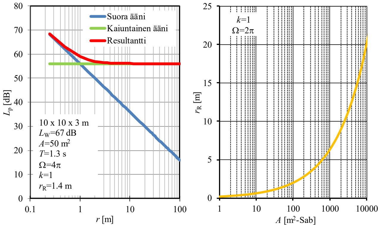
Kuva 4.3.1 (a) Suoran äänen, kaiuntaisen äänen ja edellisten resultantin äänenpainetaso L_p äänilähteen etäisyyden r funktiona eräässä huoneessa. (b) Huonepinnalle sijoitetun ympärisäteilevän äänilähteen kaiuntasäde r_R huoneen absorptioalan A funktiona. Kummatkin kuvat riippuvat taajuudesta, koska A riippuu taajuudesta.
