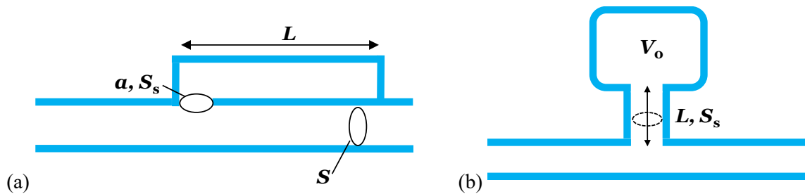
Kuva 7.19.2 (a) Neljännesaaltoresonaattori. (b) Helmholtz -resonaattori.
