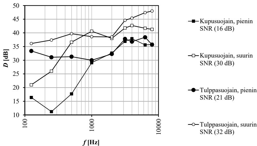
Kuva 9.2.1. Erään tuotevalmistajan pienimmän ja suurimman vaimennuskyvyn omaavien tuotteiden taajuusriippuvat suojaustehokkuusarvot.
