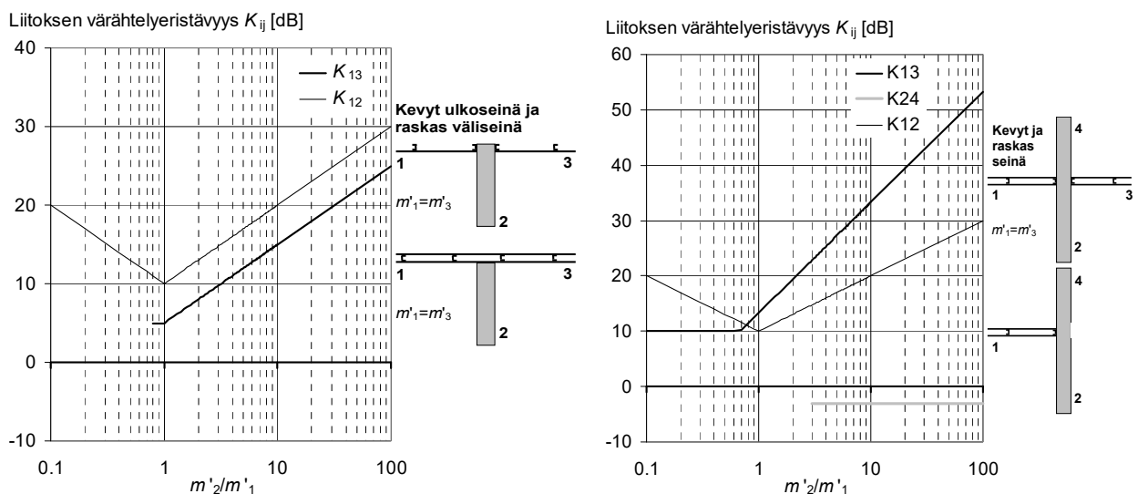
Kuva 8.3.1. Kevyen ja raskaan rakenteen liitosääneneristävyyksiä.
