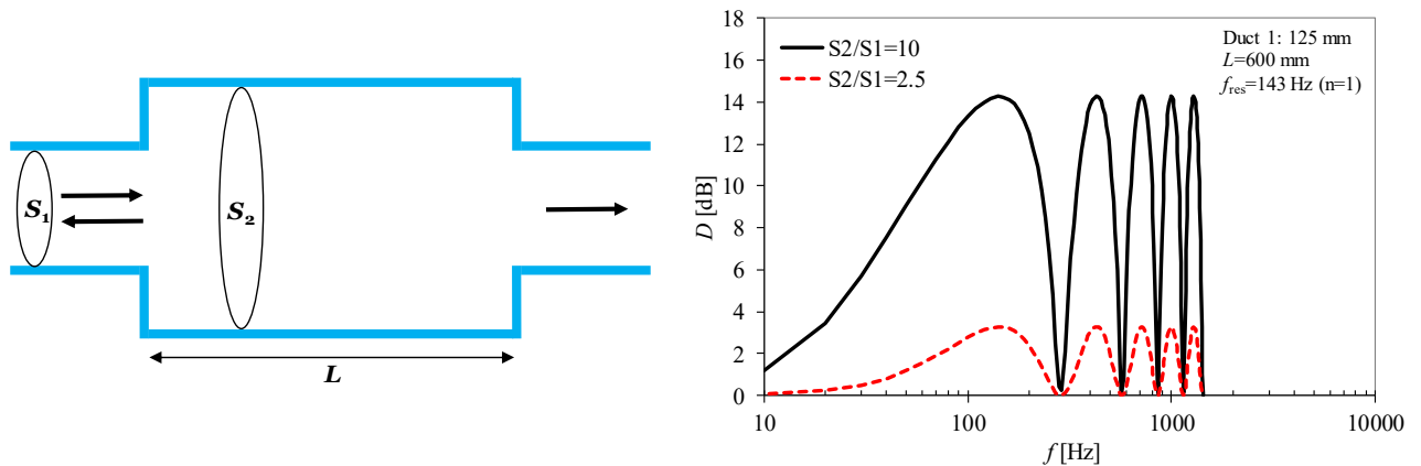
Kuva 7.19.1 (a) Kammiovaimennin ja (b) esimerkki sen äänenvaimennuksesta.
