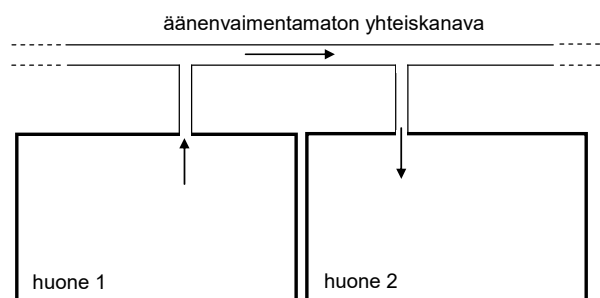
Kuva 8.9.1. Ilmanvaihtokanaviston kautta tapahtuva äänen siirtyminen tilojen välillä. Esimerkissä ei ole päätelaitteita,
