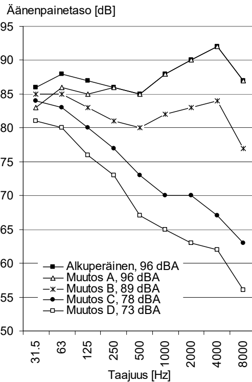
Kuva 10.6.2. Tyypillisesti saavutettavia melunvaimennuksia erilaisilla koneen ja koteloinnin järjestelyillä.
