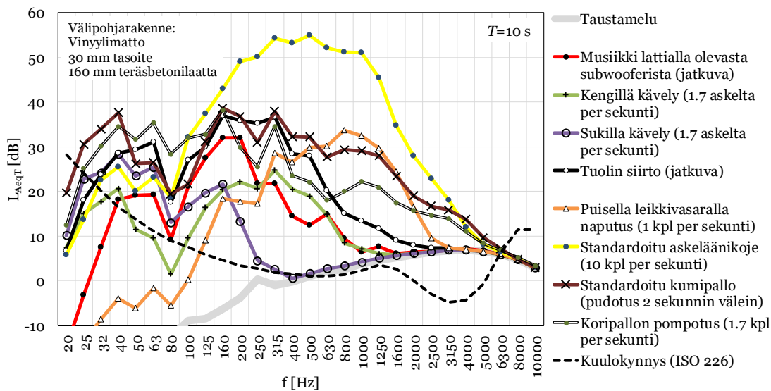
Kuva 6.6.1 Välipohjarakenteen yläpintaan kohdistuneiden iskuäänen ekvivalentteja A-painotettuja äänenpainetasoja alapuoleisessa huoneessa. Kuulokynnyksen ylittävät äänet ovat aistittavia. Impulsiivisten askeläänten kuulumista tulee siksi arvioida Fast-aikapainotetun maksimiarvon avulla. Todellisten iskuäänten äänenpainetasoille ei ole ohjearvoja, joten niillä on vain tutkimuksellista merkitystä.
