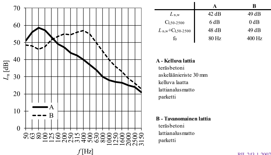
Kuva 6.2.2 Spektripainotustermin C_{1,50-2500} käytös kahdella erityyppisellä välipohjalla.
