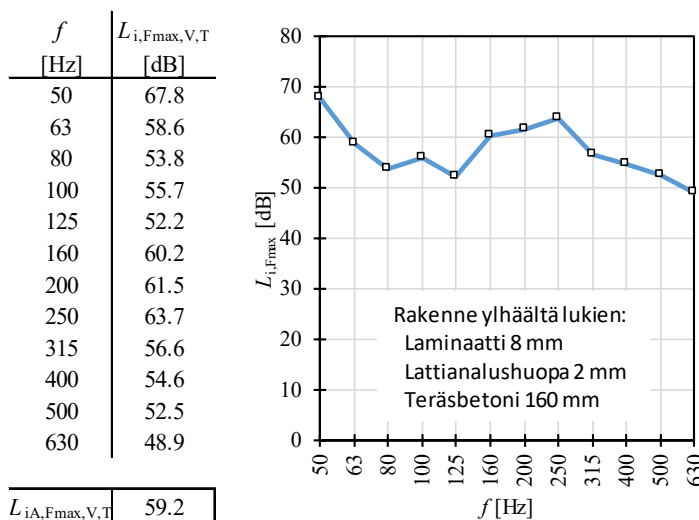
Kuva 6.6.2 Kumipallolla saatu mittaustulos hyvin tavanomaiselle 50-luvun betonivälipohjarakenteelle.
