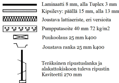
Kuva 6.5.5. Kuvissa 6.7.1–6.7.4 käytettyjen rakennekerrosten selitykset.
