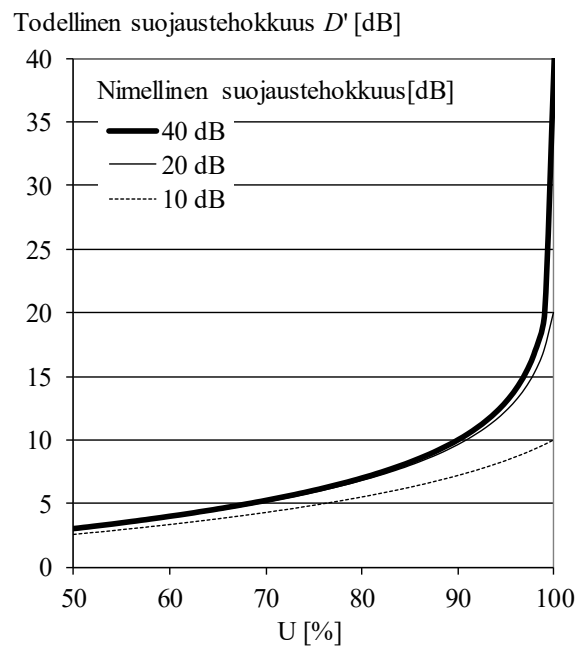
Kuva 9.4.1. Kuulonsuojaimen käyttöasteen U [% altistusajasta] vaikutus todelliseen suojaustehokkuuteen.
