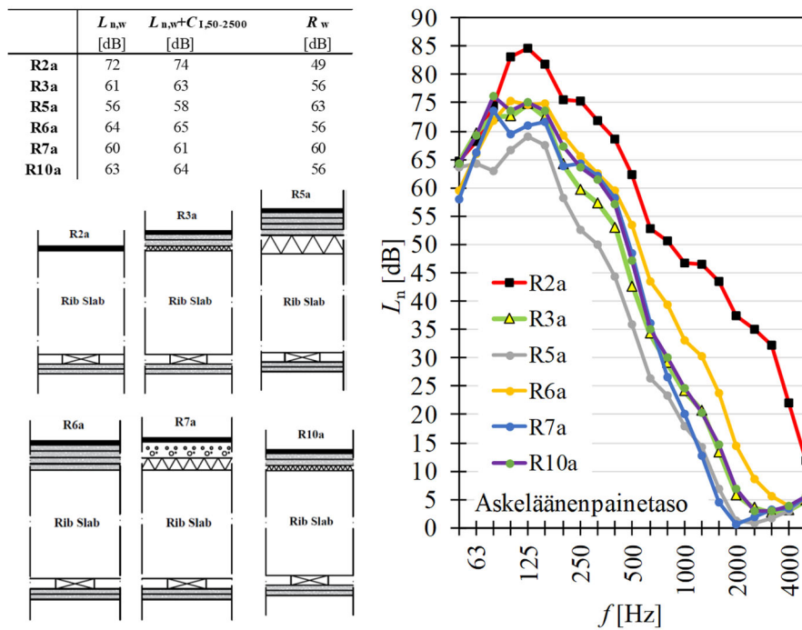
Kuva 6.7.3. Normalisoitu askeläänenpainetaso taajuuden funktiona, kun kantava rakenne on 370 mm paksu puinen avokotelolaatta (Rib Slab) jäykästi koolatulla alakatolla ja laatan päällysteisiin kohdistuu muutoksia.
