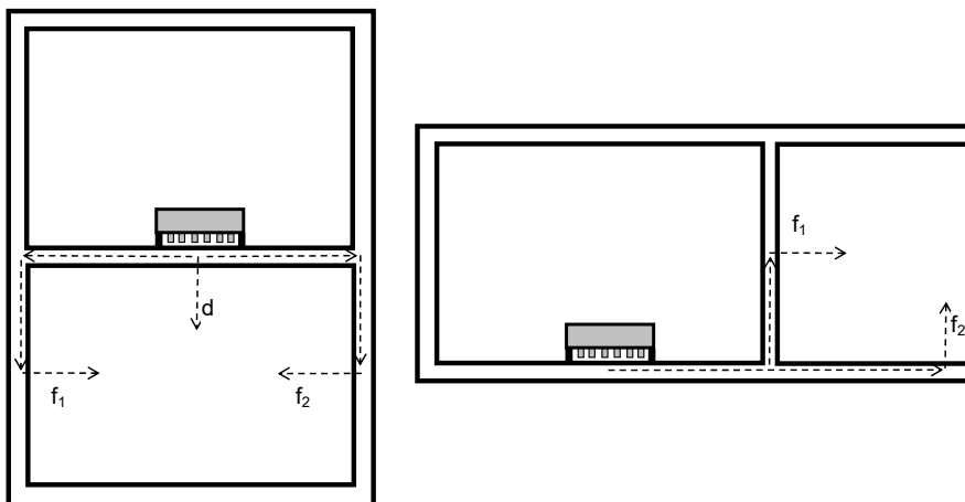
Kuva 8.4.1. Pystysuuntaisen ja vaakasuuntaisen askeläänenpainetaso muodostuminen 2 dimensiossa.
