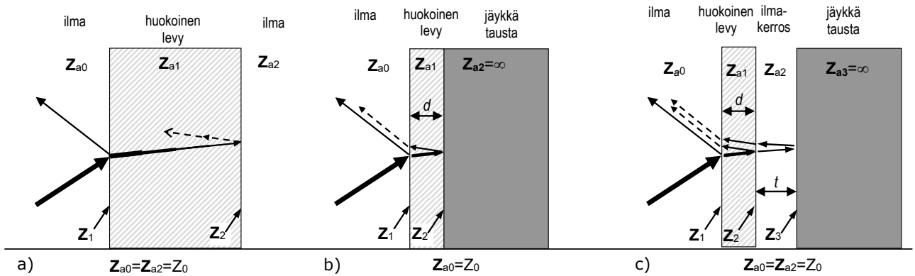
Kuva 3.6.1. Kolme huokoisen levyn asennustapaa. Huokoinen levy on merkitty vaaleanharmaalla ja tummanharmaa materiaali on suuri-impedanssinen, täysin heijastava taustaseinä.
