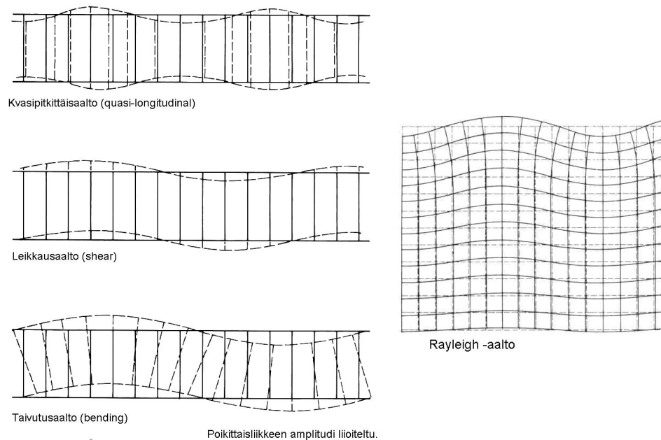
Kuva 5.3.1 Vasemmalla on esitetty levyssä etenevät merkittävät aaltomuodot (Lähde: Fahy 1985). Oikealla on kuva Rayleighin pinta-aalloista, kun materiaali on ylhäällä. (Lähde: Cremer and Heckl, 1988).
