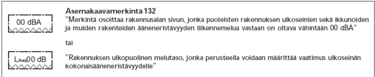
Kuva 8.8.1. Kaavamerkintöjä. Ylempi merkintä on ulko- ja sisämelutason erotus, \Delta L , ja alempi on ulkomelutaso L_{A,eq,u} .
