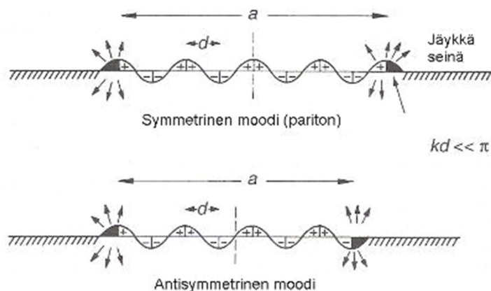
Kuva 5.6.2 Akustinen oikosulku reunamoodin tapauksessa, kun f < \frac{1}{2}f_c . Kuvassa a on levyn mitta tarkasteltavan akselin suunnassa. Oikosulun vuoksi levyn lähikentässä on pyörteisyyttä eikä esimerkiksi intensiteettimittauksia sen vuoksi suositella tehtävän alle 10 cm päässä pinnasta (Lähde: Fahy 1985).
