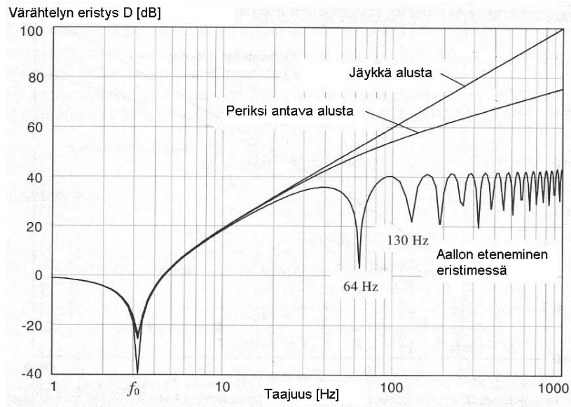
Kuva 11.6.2. Käytännössä värinäeristys kasvaa harvoin yli 30 dB:n, koska eristimessä on resonansseja. (Boden et al., 1999)
