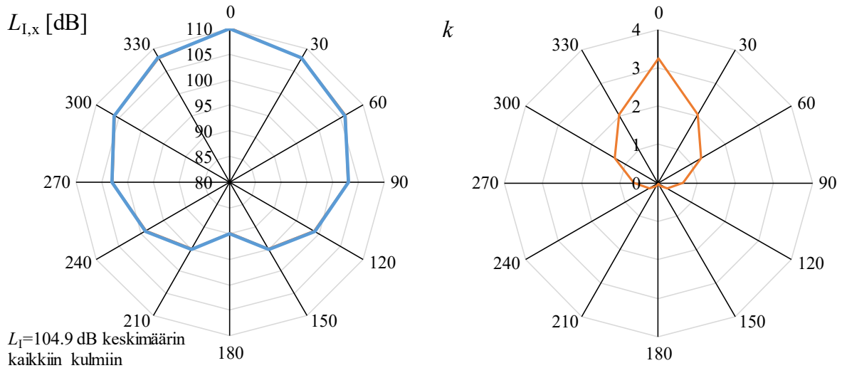
Kuva 2.4.1. Erään äänilähteen suuntaavuusominaisuuksia horisontaalitasossa 30 asteen välein. Vasemmalla intensiteettitaso L_{I,x} eri kulmilla x . Oikealla edellisestä johdettu suuntakerroin k eri kulmilla. Kulmassa 0^\circ on k=3.25 ja L_k=5.1 dB.
