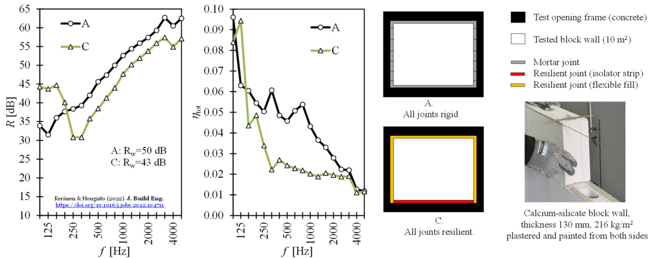
Kuva 5.7.2 Harkkoseinän ilmapääeneristävyyden, R , ja kokonaishäviökerroin, \eta_{tot} , taajuuden, f , funktiona, kun harkkoseinän liitokset ovat jäykät (A) tai elastiset (B). Jäykkä asennustapa on tavanomainen (Keränen & Hongisto, 2022).
