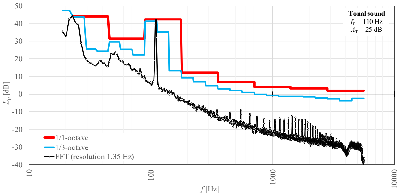
Kuva 1.4.2 Eräästä tonaalisesta äänestä tehty FFT-, terssikaista- ja oktaavikaista-analyysi.
