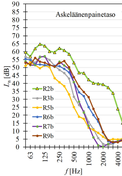
Kuva 6.7.4. Normalisoitu askeläänepainetaso taajuuden funktiona, kun kantava rakenne on 370 mm paksu puinen avokotelolaatta (Rib Slab) joustavasti koolatulla alakatolla ja laatan päällysteisiin kohdistuu muutoksia.
