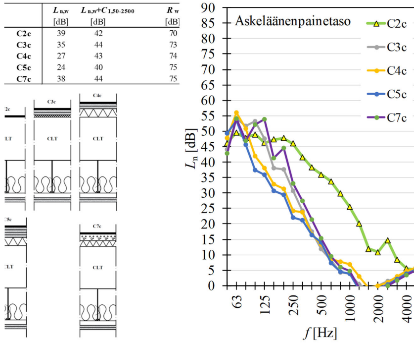
Kuva 6.7.2. Normalisoitu askeläänenpainetaso taajuuden funktiona, kun kantava rakenne on 260 mm paksu massiivipuulaatta (CLT) ripustuslanka-alakatolla ja laatan päällysteisiin kohdistuu muutoksia.
