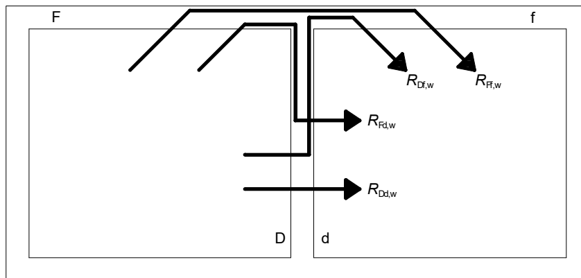
Kuva 8.2.3. Sivutiesiirtymäreittien merkintätavat EN 12354-1 mukaan yhdelle sivuavalle rakenteelle. Lähetys huone on vasemmalla ja vastaanottohuone oikealla.
