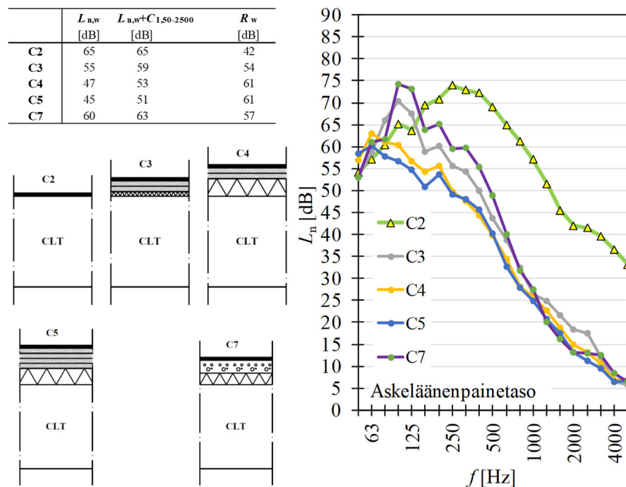
Kuva 6.7.1. Normalisoitu askeläänepainetaso taajuuden funktiona, kun kantava rakenne on 260 mm paksu massiivipuulaatta (CLT) ja laatan päällysteisiin kohdistuu muutoksia.
