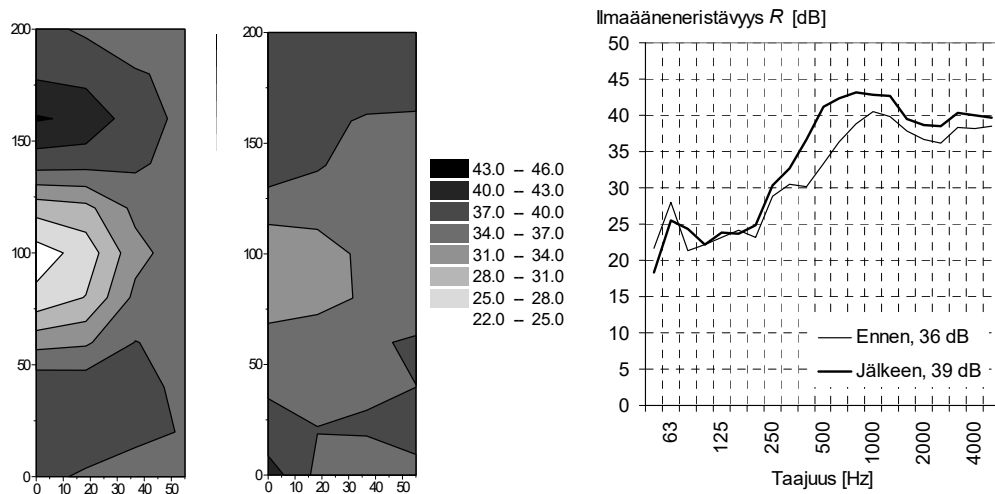
Kuva 5.1.1 Erään ovirakenteen ilmaääneneristävyys ennen ja jälkeen oven lukon tiivistyksen taajuudella 500 Hz. Värit kertovat karkeasti paikallisesta ilmaääneneristävydestä [dB]. Oikealla on esitetty ilmaääneneristävyys. Ennen: tiivistämätön lukko. Jälkeen: tiivistetty lukko. R_w -arvojen ero oli 3 dB.
