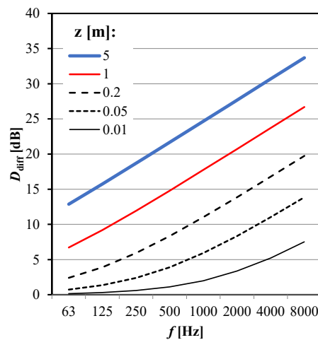
Kuva 2.9.2. Melusteellä tiettyyn tarkastelupisteeseen aikaansaadun matkaeron z [m] vaikutus äänenvaimennukseen eri taajuuksilla olettaen, että meluesteen läpi tai ohi ei kulkeudu ääntä.
