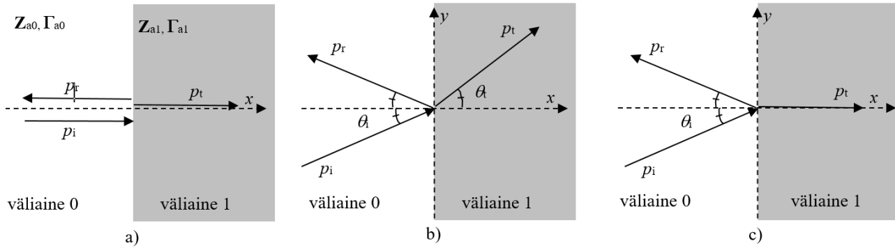
Kuva 3.3.1 Heijastuminen ja läpäisy kahden materiaalin rajapinnassa. a) Kohtisuora tulokulma, \theta = 0^\circ . (b) Vinko tulokulma ja kokonaisuutena reagoiva materiaali (läpäisykulma \theta riippuu äänen nopeudesta väliaineessa 1). (c) Vinko tulokulma ja paikallisesti reagoiva materiaali (läpäisykulma on aina 0^\circ ).
