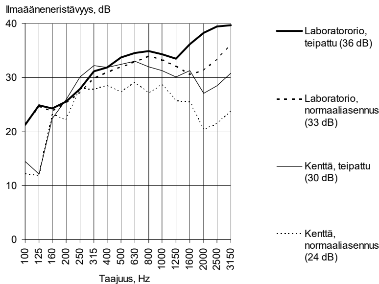
Kuva 8.7.1. Erään desibelioiven (oviluokka 30 dB) ilmääneneristävyys laboratoriossa ja kentällä rakennuskohteessa. Mittaus tehtiin normaaliasennuksen lisäksi saumat teipattuna, jolloin nähdään vuotojen osuus. Sulkeissa R_w / R'_w -arvot.
