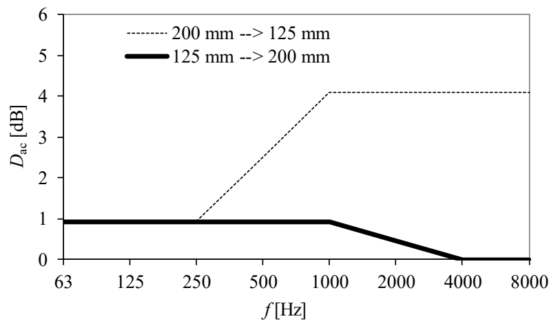
Kuva 7.13.2 Äänenvaimennus pyöreän ilmanvaihdon kanavan yhtäkkisessä muutoskohdassa, kun kanava pienenee (ohut viiva) tai kasvaa (paksu viiva). Mitat ovat kanavahalkaisijoita.
