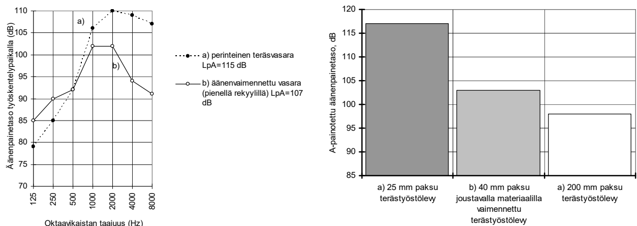
Kuva 10.5.1. Esimerkkejä vasaroinnin meluntorjunnasta vasaratyyppiä vaihtamalla tai työstettävän kohtion massaa kasvattamalla.
