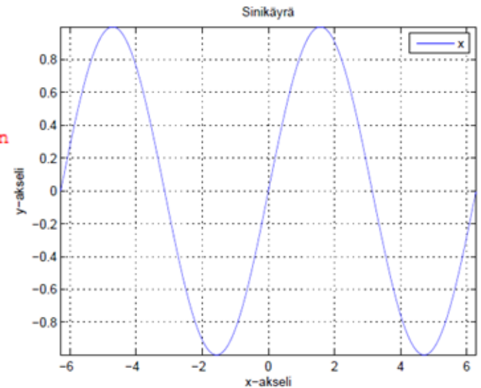
Figure 1: Funktion \sin(x) kuvaaja
