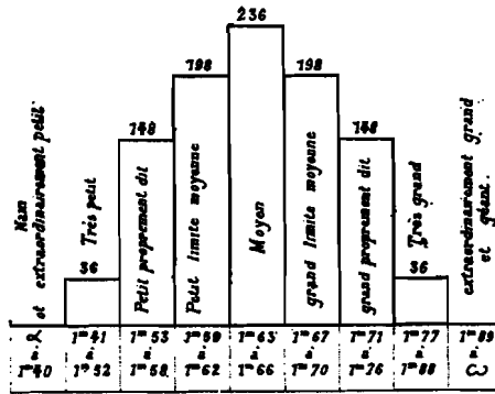
Fig. 5. — DIAGRAMME DE LA TAILLE INDICANT PAR LA HAUTEUR PROPORTIONNELLE DES COLONNES LE NOMBRE DES SUJETS REMPLISSANT À CHACUNE DES SEPT CATÉGORIES DE TAILLE INDICÉES SUR LA COURBE BINOMIALE (Fig. 4).
