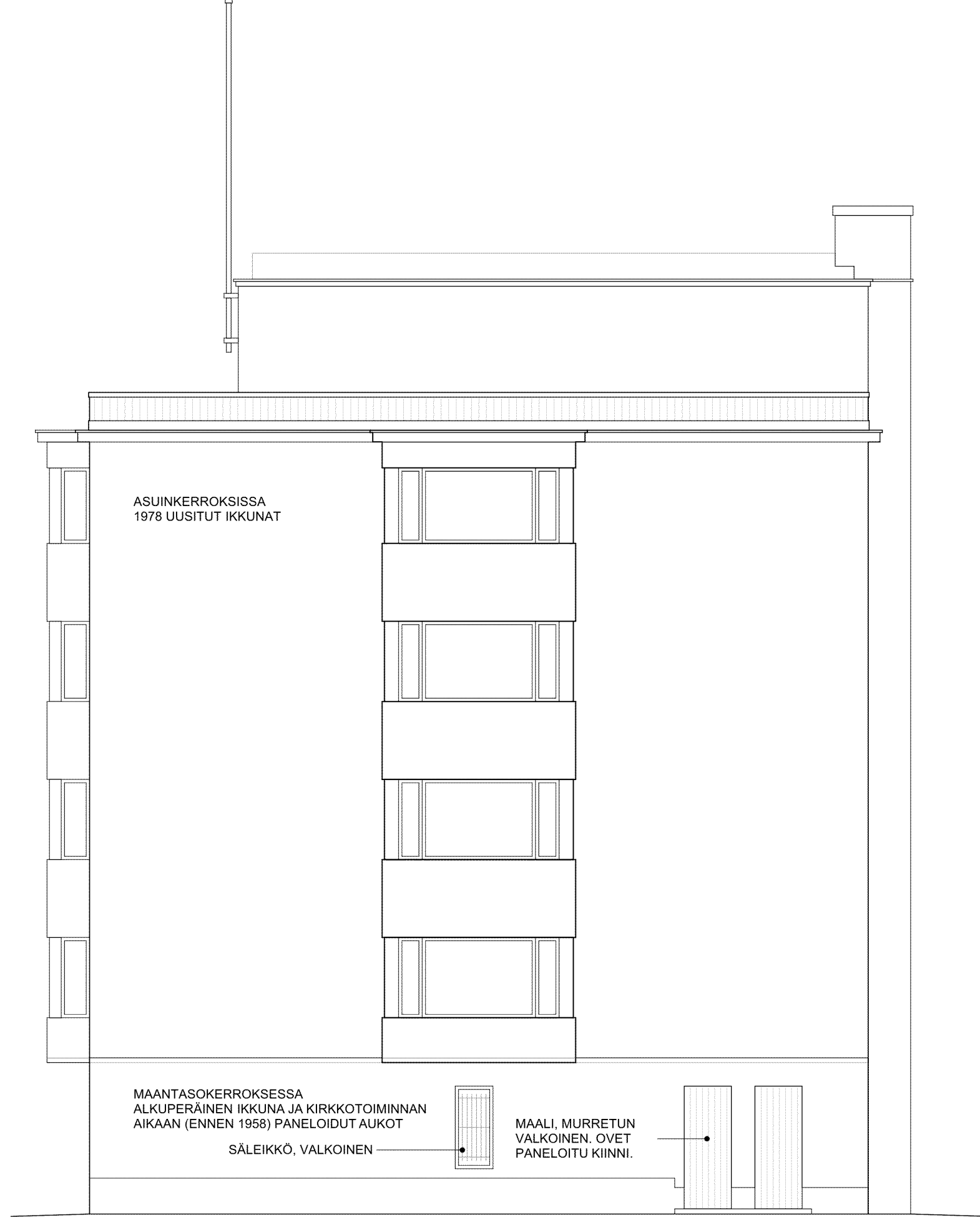
JULKISIVU LÄNTEEN
