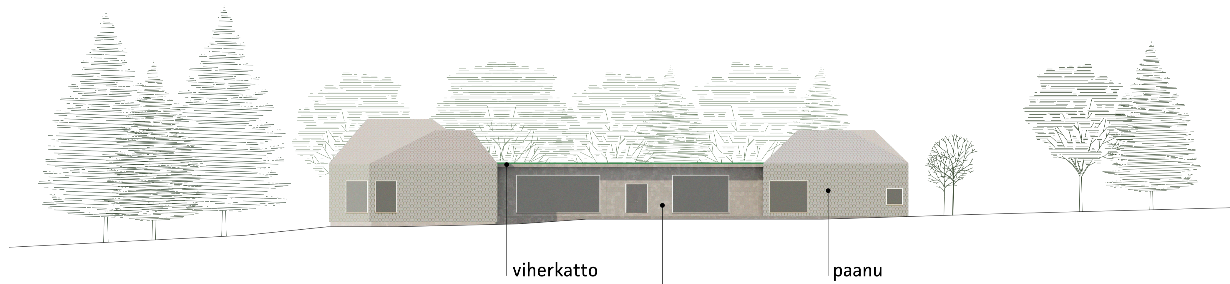
julkisivu lounaaseen 1:200
