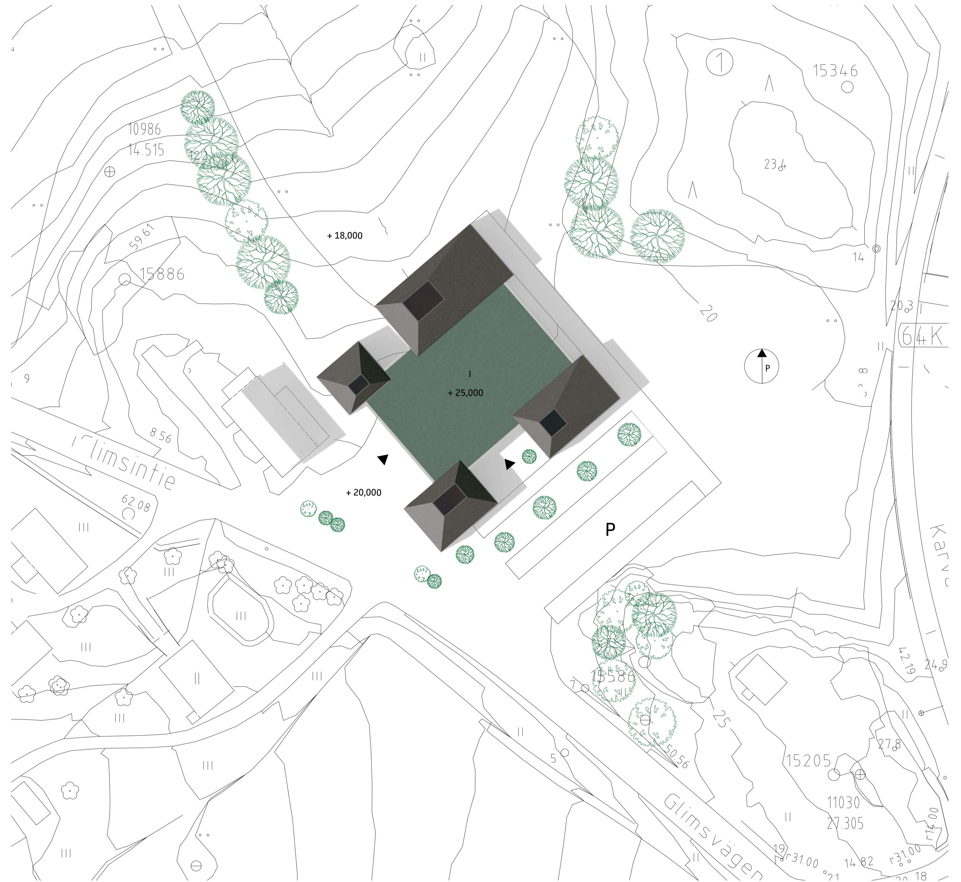
asemapiirustus 1:500
