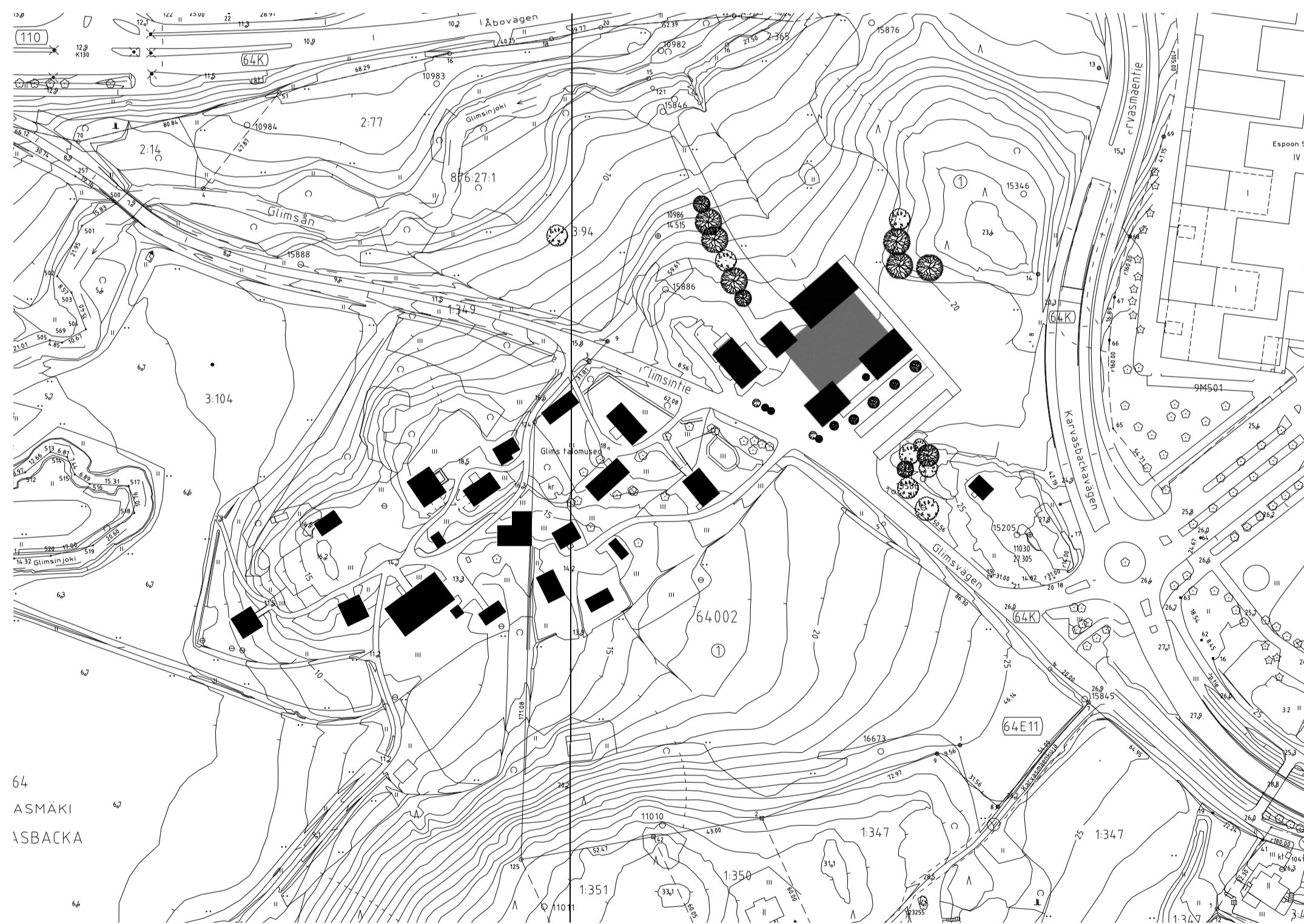
liittyminen ympäristöön 1:2000
